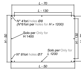
Vista pannello di cablaggio Wiring panel view
